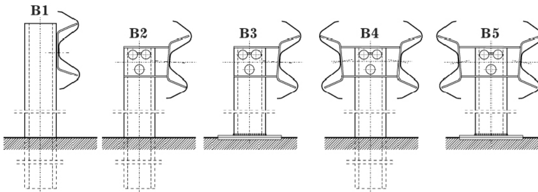
Ограда со одстојник за објекти (сите елементи се топло поцинкувани)
