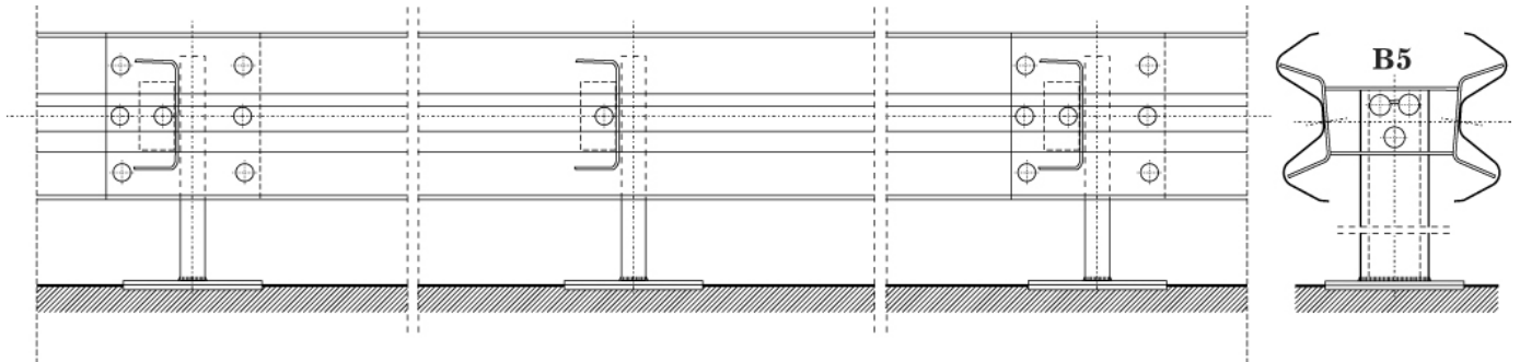
Ограда со одстојник за објекти (сите елементи се топло поцинкувани)
